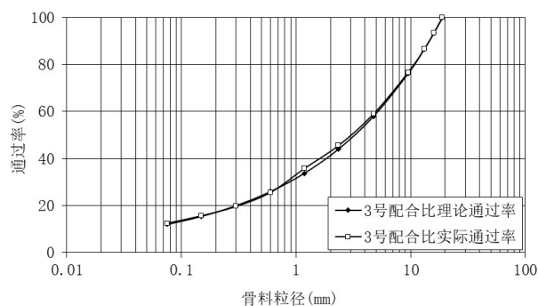
图2 沥青混凝土骨料粒径与累计通过率分布
