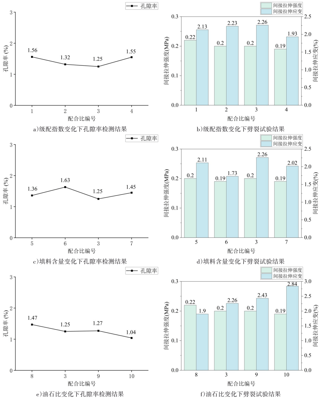
图1 孔隙率检测和劈裂试验结果
